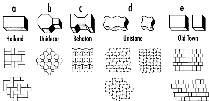
Rys. 2. Najczęściej spotykane kształty kostek i sposoby (desenie) ich układania (wg W. Brylicki: Kostka brukowa z betonu wibroprasowanego, 1998)
