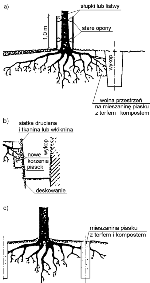
Rys. 2. Zabezpieczenie drzew przy obniżeniu terenu, po wykonaniu wykopów (wg N.P. Ornatski: Drogi i ochrona przyrody, Transport 1982)
