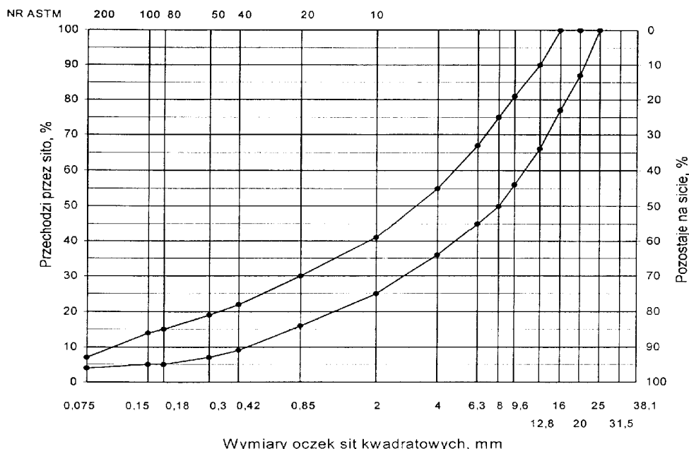
Rys. 12. Krzywe graniczne uziarnienia mieszkanki mineralnej BA od 0 do 20 mm do warstwy wiążącej, wyrównawczej i wzmacniającej nawierzchni drogi o obciążeniu ruchem od KR3 do KR6
