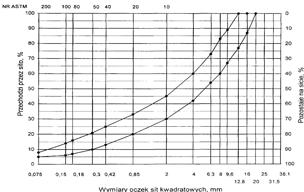
Rys. 13. Krzywe graniczne uziarnienia mieszkanki mineralnej BA od 0 do 16 mm do warstwy wyrównawczej nawierzchni drogi o obciążeniu ruchem od KR3 do KR6
